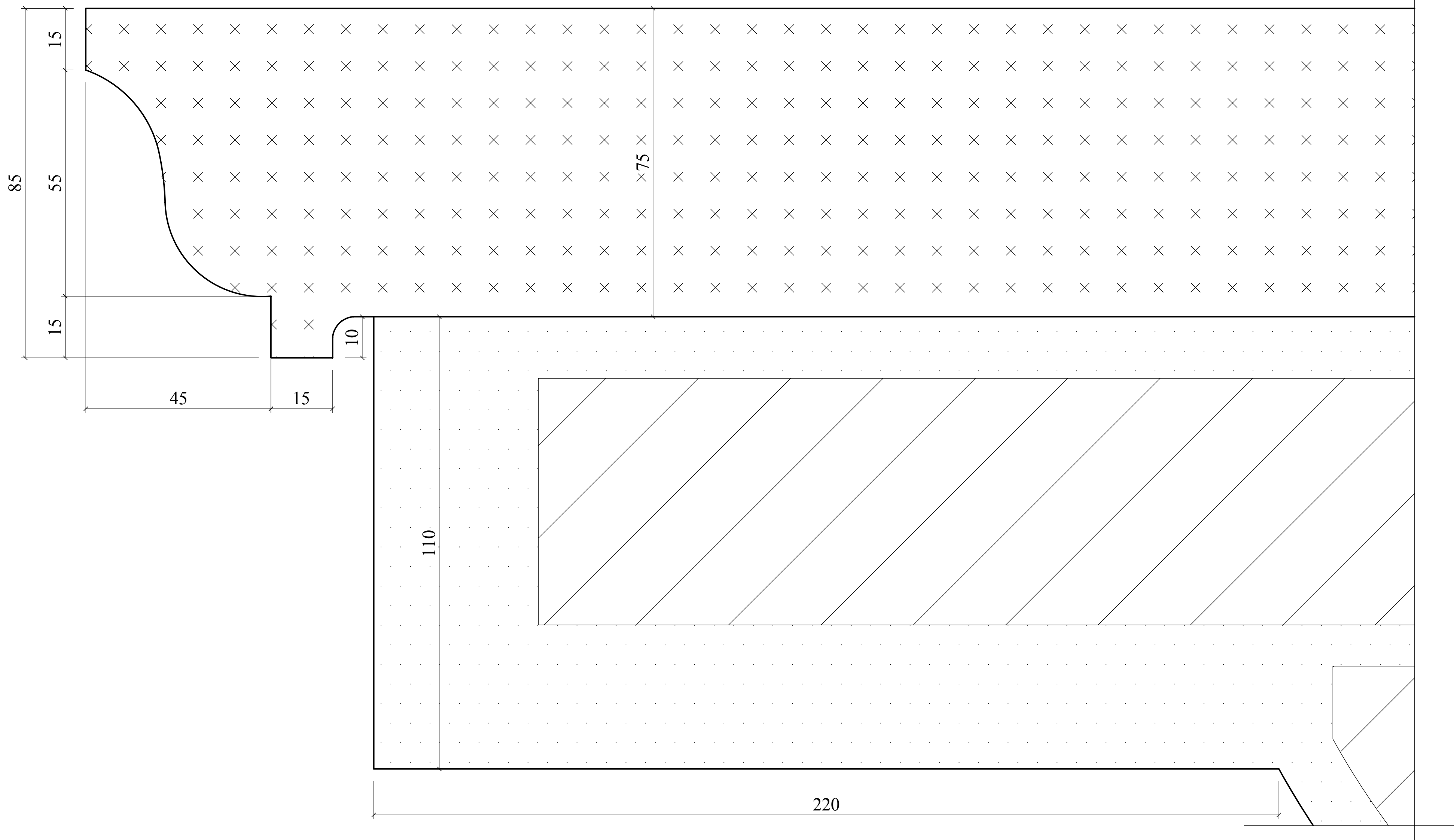
Gzyms z piaskowca , skala 1 : 1
